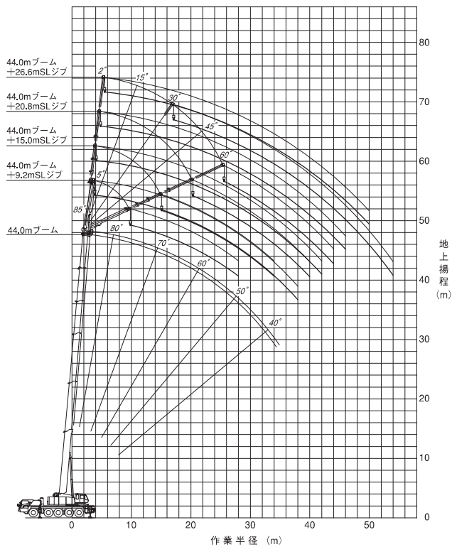
スーパーラフィングジブ (SLジブ) 作業範囲図 【44.0mブーム+9.2m~26.6mSLジブ】
