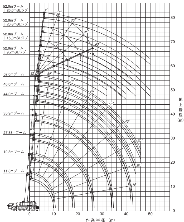
スーパーラフィングジブ (SLジブ) 作業範囲図 【52.0mブーム+9.2m~26.6mSLジブ】
