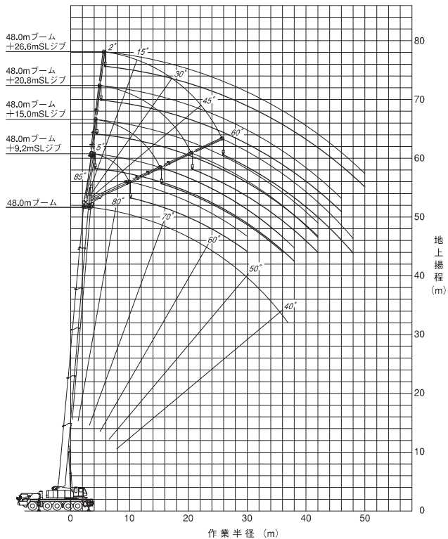
スーパーラフィングジブ (SLジブ) 作業範囲図 【48.0mブーム+9.2m~26.6mSLジブ】
