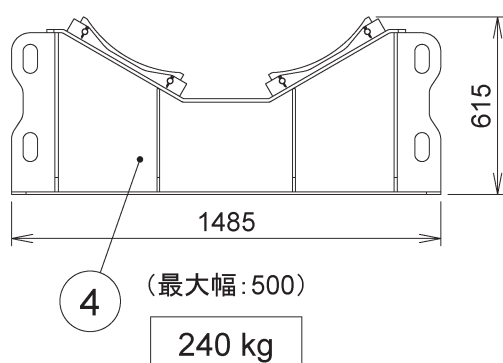
ブーム輸送用スタンド
