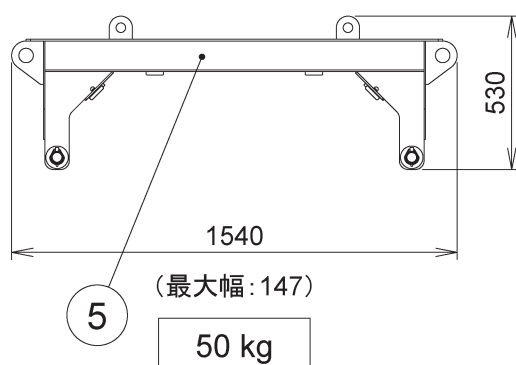
ブーム輸送用固定ハンガー
