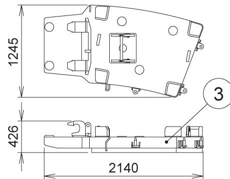
3 ton サイドベースウェイト(右)
