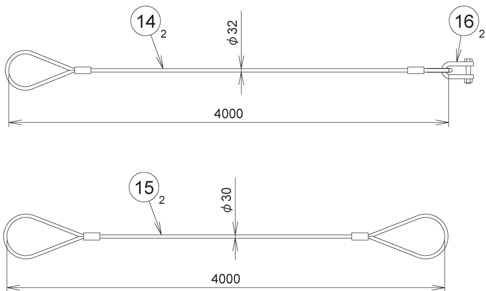
カウンターウエイト用吊りロープ
